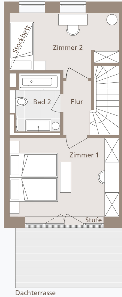
Staffelgeschoss
